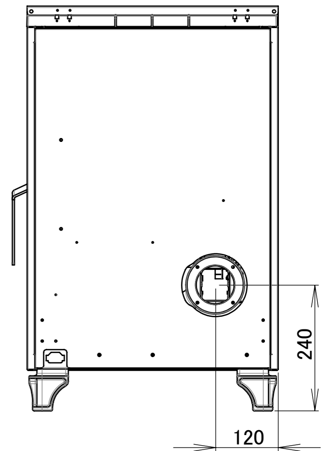
SAIKAI SS-5 外觀寸法図
