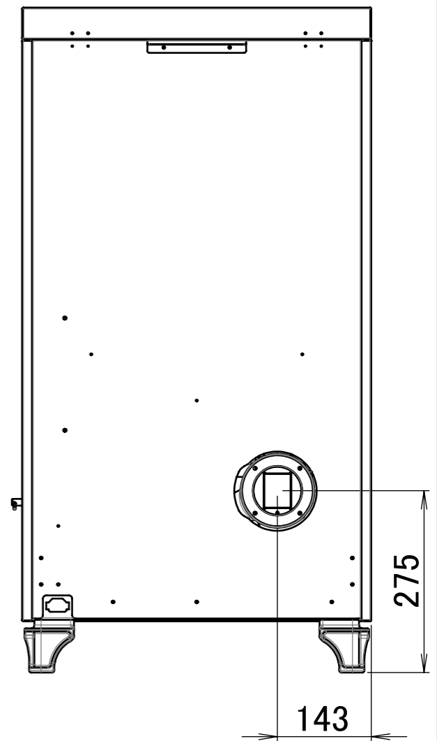
SAIKAI SS-10 外觀寸法図
